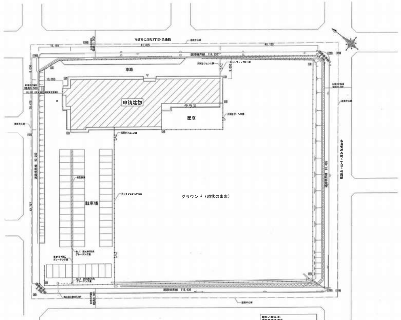
配置図 S-1/300
