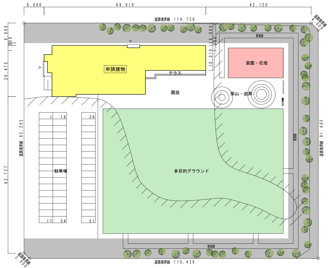
配置図 S = 1 / 500
